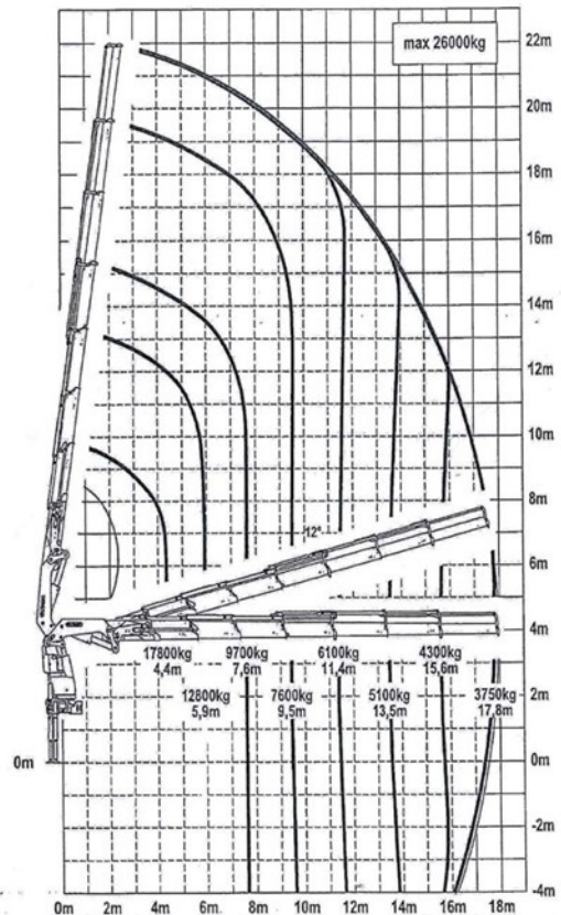
020.06200 PK 92002 SH Traglastdiagramm PK 92002-SH F
